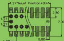
3524-383XXMXX064X1
