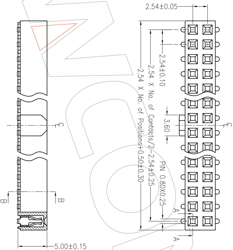
Section A-A
