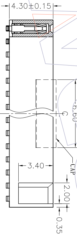
SECTION A-A
